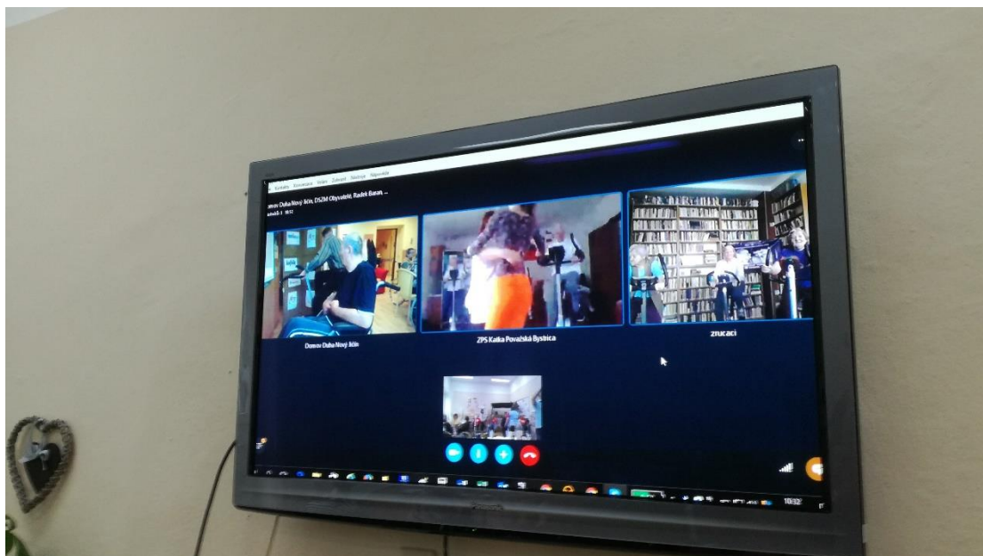
Obr. 2 Skype komunikace
